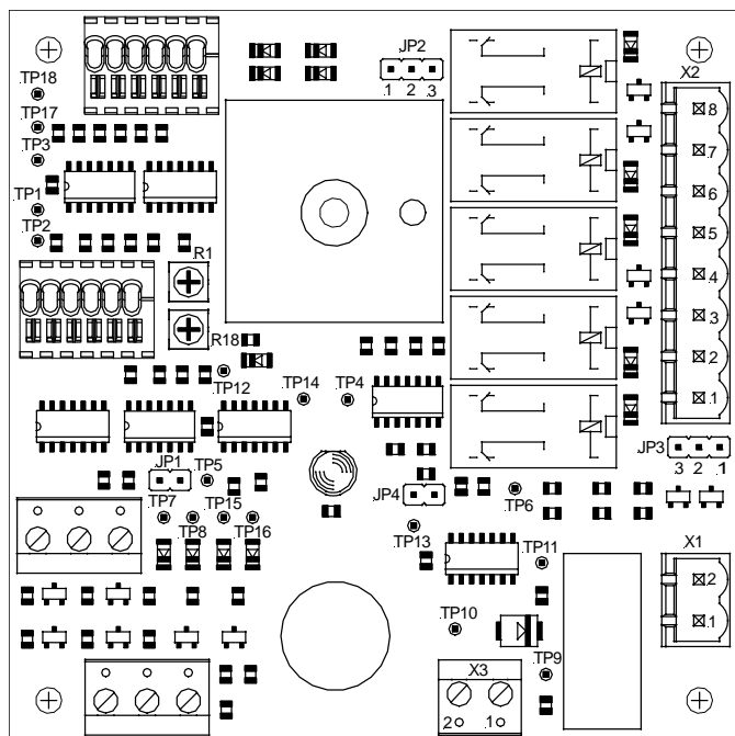
Abb. 2 – Lage der Anschlüsse, Testpunkte und Einstellmöglichkeiten
